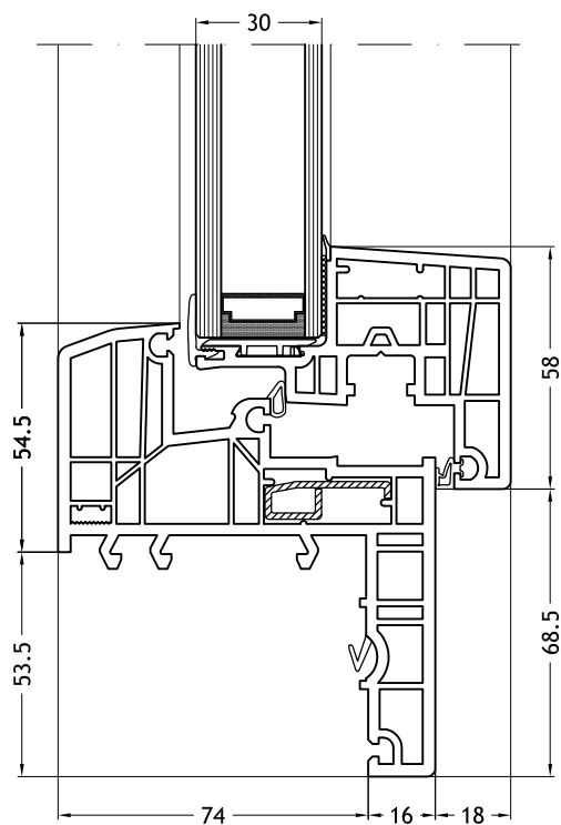
Soglia ribassata con anta Nova-line 971
