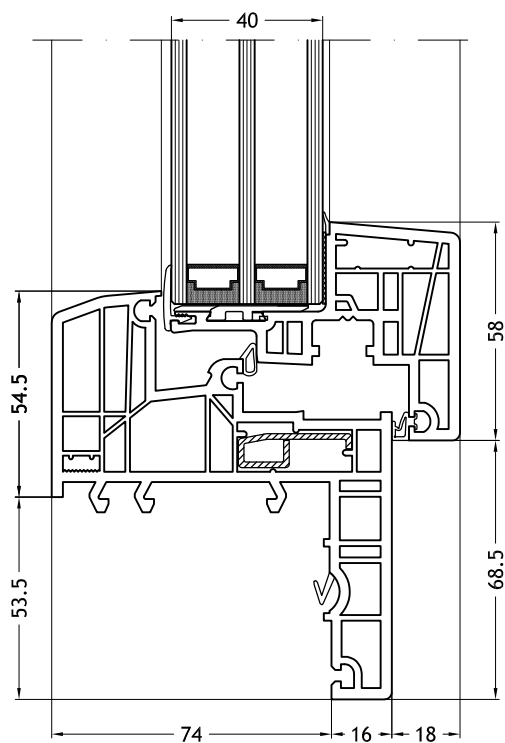
Soglia ribassata con anta Nova-line 953
