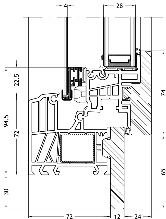
Telaio a Z 9C60 con anta Nova-line Twin
