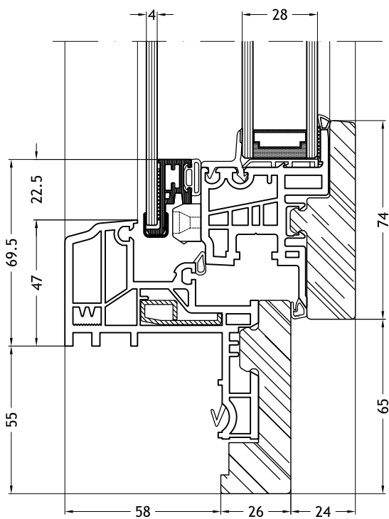
Telaio a Z 9D163 con anta Nova-line Twin
