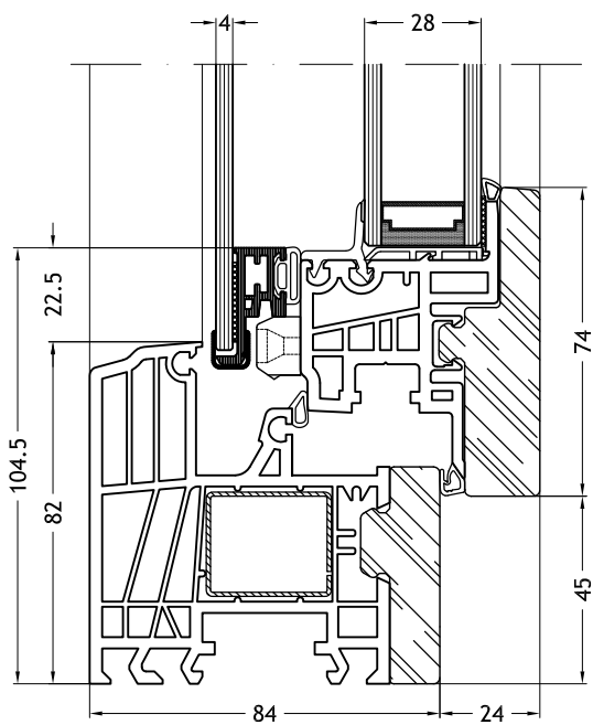
Telaio a L 9B43 con anta Nova-line Twin
