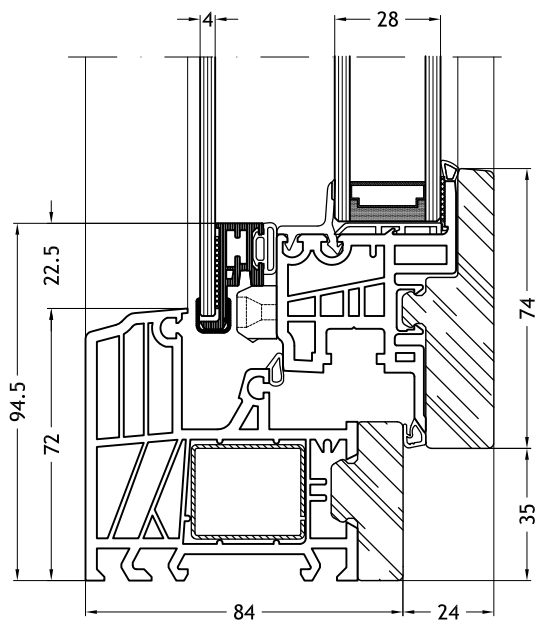
Telaio a L 9A60 con anta Nova-line Twin
