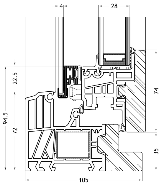
Telaio a L 9F60 con anta Nova-line Twin
