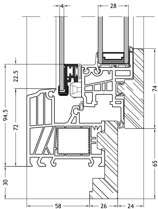
Telaio a Z 9D60 con anta Nova-line Twin
