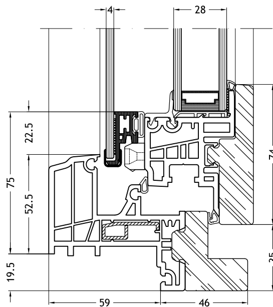
Telaio a Z 9F136 con anta Nova-line Twin
