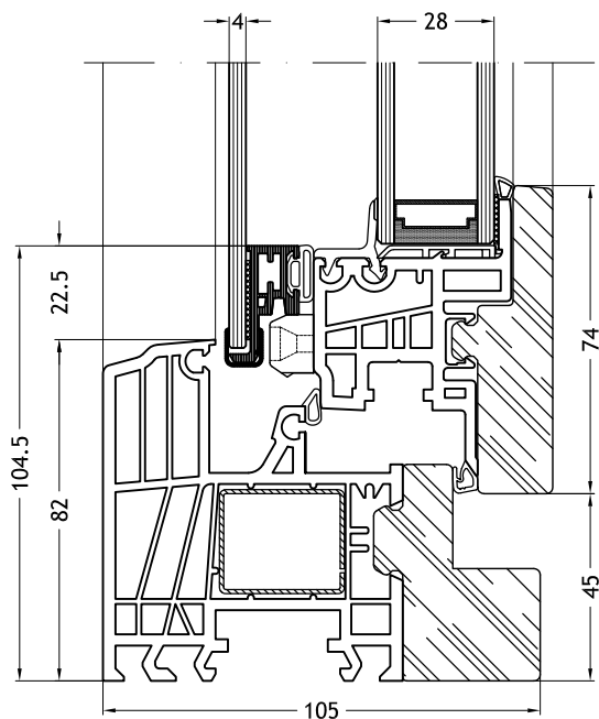
Telaio a L 9G43 con anta Nova-line Twin
