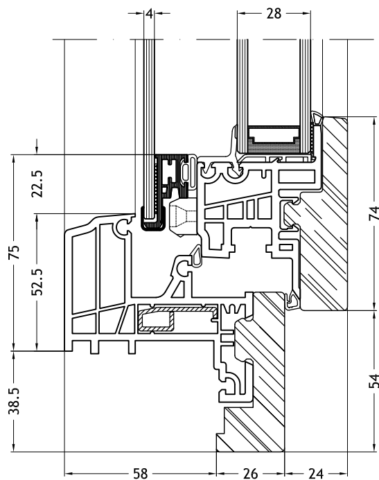
Telaio a Z 9E136 con anta Nova-line Twin
