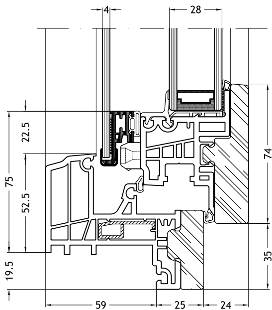
Telaio a Z 9A136 con anta Nova-line Twin
